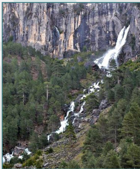
Los "Merguizos" del Aguamula (Santiago-Pontones, Jaén), uno de los "reventones" más espectaculares y efímeros que conozco. Corresponden al nacimiento de "aguas altas" del río Aguamula, en la sierra de Segura (foto Luis Cano)
